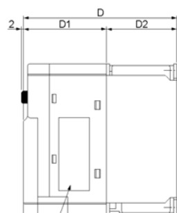
Plaque signalétique
